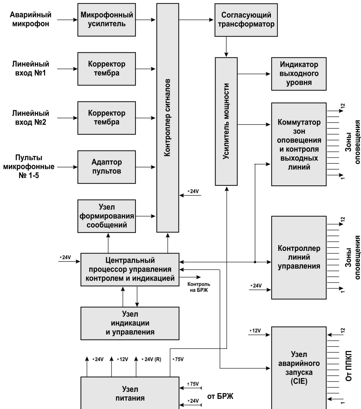
Рисунок 2 - Структурная схема блока
