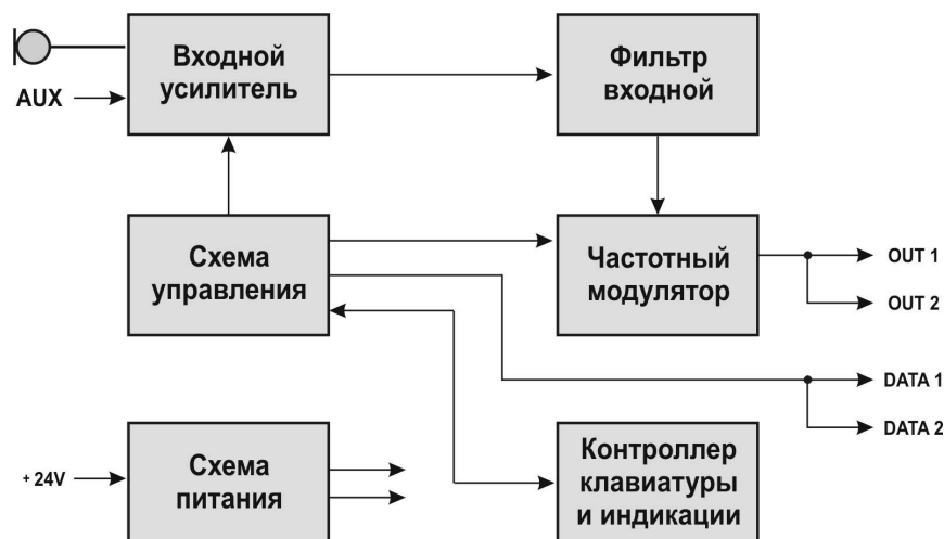
Рисунок 4 - Структурная схема пульта микрофонного
