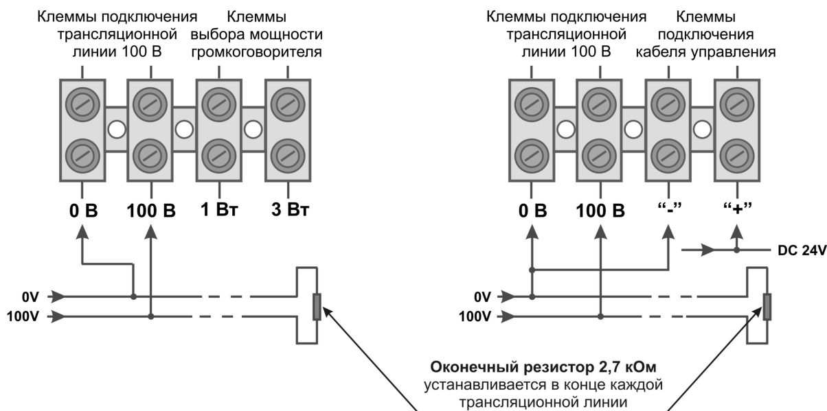
Схема подключения громкоговорителя к трансляционной линии
