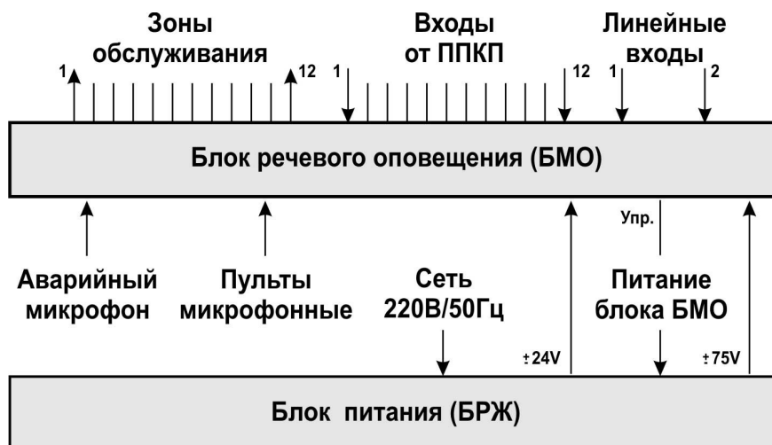
Рисунок 1 - Структурная схема оборудования
