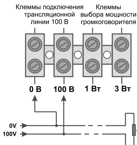
Схема подключения громкоговорителя к трансляционной линии
