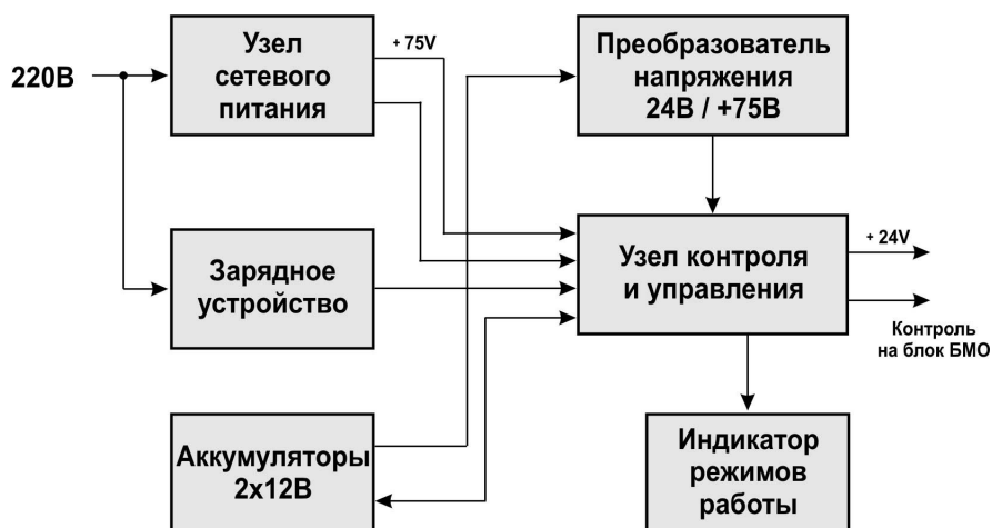
Рисунок 3 - Структурная схема блока
